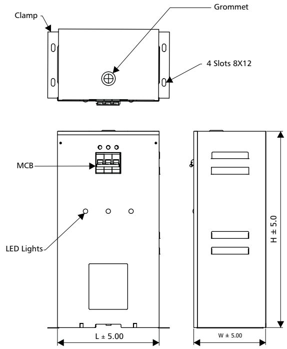
20 to 25 kVAr
